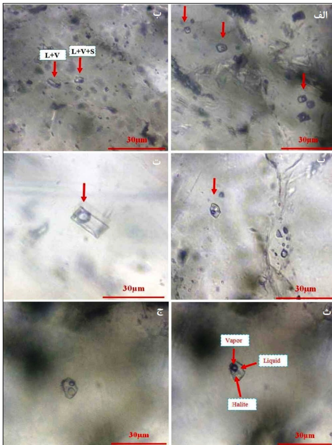
شکل ۸ (الف) نمایی از میانبرهای شاری دو فازگی غنی از مایع (L+V). (ب) دو نوع میانبار بررسی شده (L+V) و (L+V+S). (پ) میانبار سه فازگی (L+V+S) به شکل بلورین منفی. (ت) میانبار دو فازگی (L+V) به شکل بلورین منفی. (ث) میانبار سه فازگی (L+V+S) متشکل از فاز گاز (V)، مایع آبگین (L) و هالیت. (ج) همان میانبار در دمای 160^{\circ}\text{C} درجه سانتی‌گراد. حاشیه‌های بلور هالیت گرد شده است.
