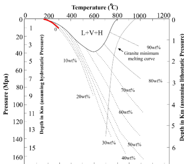
شکل ۱۰ نمودار فشار- دمای نشان‌دهنده رابطه فازها در سامانه H_2O-NaCl در فشارهای هیدرواستاتی و سنگ ایستایی [۲۵]. L = مایع، V = بخار، H = حالت. خط‌چین‌ها پربندهای ثابت درصد وزنی NaCl محلول در شورا به هستند. خط باریک خاکستری منحنی کمترین ذوب گرانیات را مشخص می‌کند. خط ضخیم مشکی مرز سه فازی، L+V+H را برای سامانه NaCl-KCl-H_2O با Na/K در محلول ثابت شده بوسیله آل‌بیت و فلدسپار قلیایی در دماهای مشخص نشان می‌دهد.
