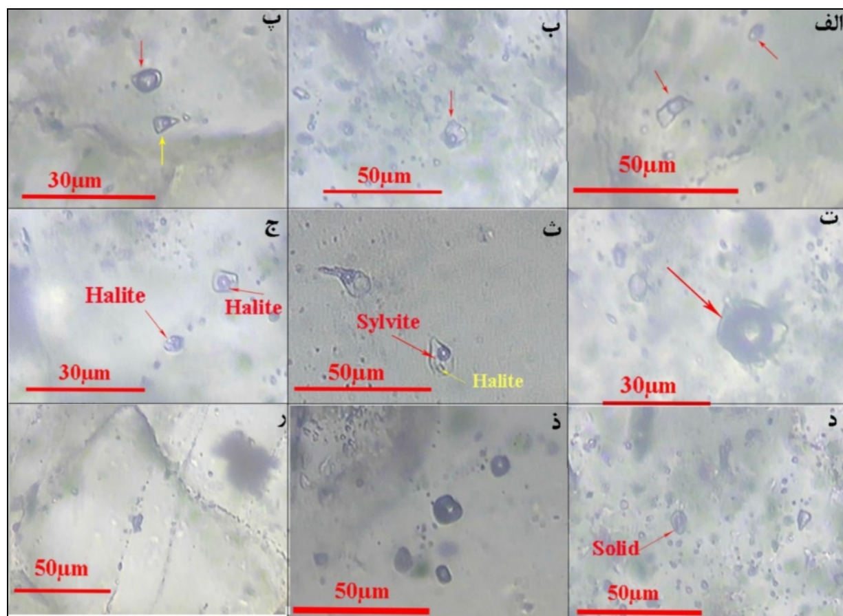
شکل ۸. نوع و شکل میانبارهای سیال الف و ب) دوفازی غنی از مایع (پیکان قرمز؛ پ) دوفازی غنی از بخار (پیکان قرمز) و دوفازی غنی از مایع (پیکان زرد؛ ت) دوفازی غنی از بخار؛ ث) میانبارهای اشباع از نمک، فازهای بخار + مایع + بلور هالیت ± سیلویت؛ ج) میانبار سه‌فازی بخار + مایع + بلور هالیت؛ چ) میانبار سه‌فازی بخار + مایع + جامد (فاز ناشناخته؛ ح) میانبارهای تک‌فاز بخار؛ خ) میانبارهای ثانویه‌ای که مرز بلوری را قطع کرده‌اند.
