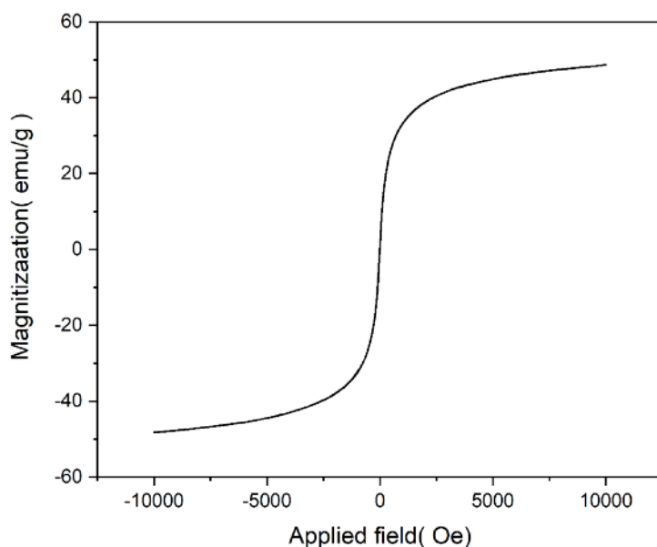
شکل ۴ الگوی VSM نانوذرات \text{Fe}_3\text{O}_4 .
