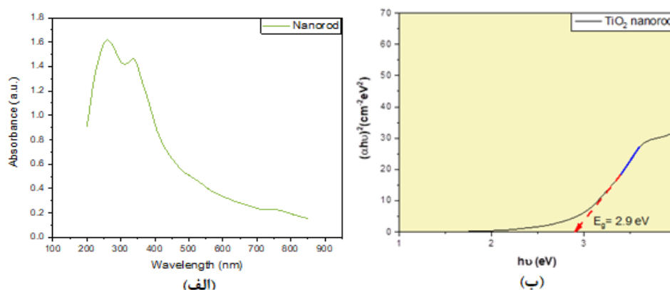
شکل ۱۵ الف) طیف جذب UV-vis نانومیله دی‌اکسید تیتانیوم و ب) نمودار تاؤک برای محاسبه گاف انرژی نانومیله دی‌اکسید تیتانیوم.
