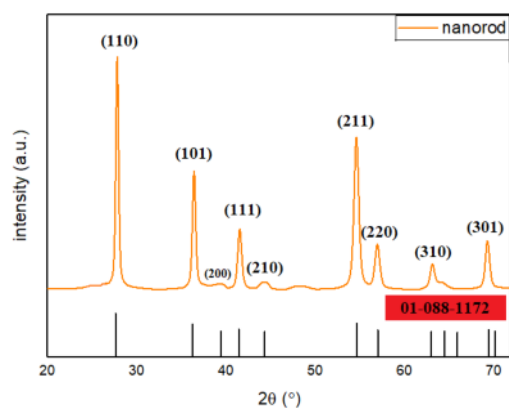
شکل ۱ الگوی پراش پرتوی ایکس نانومیله‌های دی‌اکسید تیتانیوم با فاز روتیل به همراه شاخص‌های میلر کارت استاندارد JCPDS.
